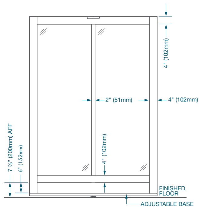
CENTER PIVOT DOOR FRAMED 4" STILE - ADA
