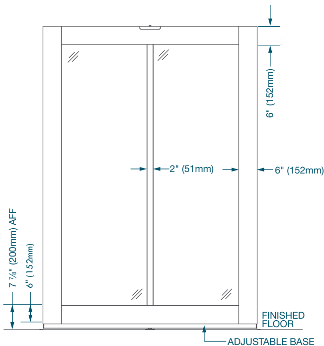
CENTER PIVOT DOOR FRAMED 6" STILE
