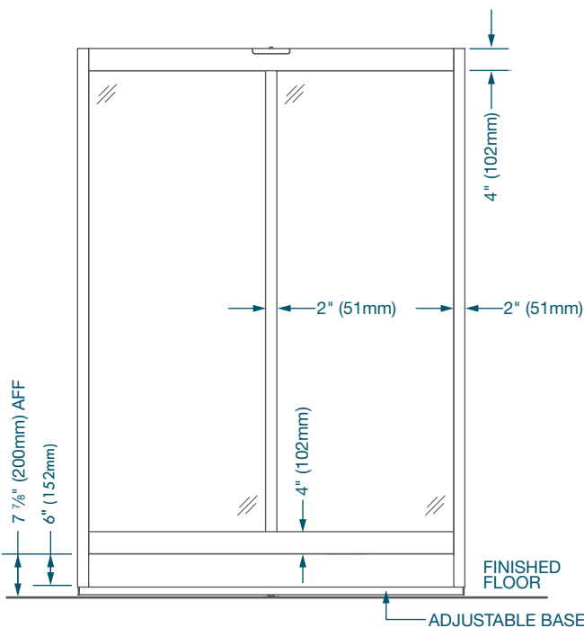
CENTER PIVOT DOOR FRAMED 2" STILE - ADA
