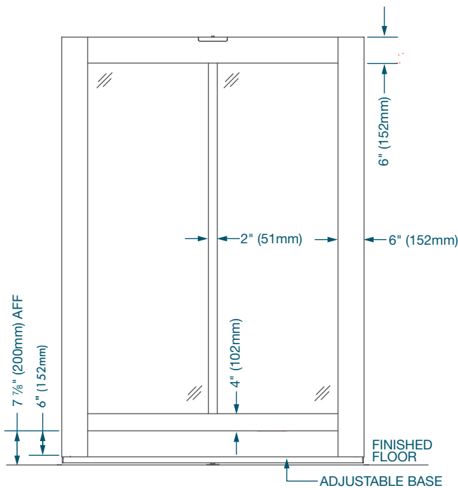
CENTER PIVOT DOOR FRAMED 6" STILE - ADA
